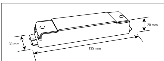
AFMETINGEN B-LDCC-10W-100-450D
